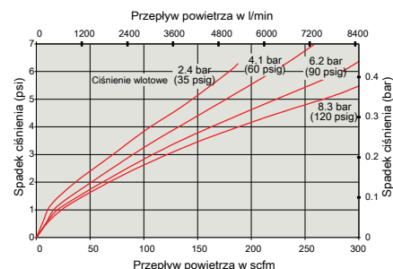
Smarownica 1"
