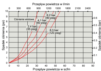
Filtr 1/4"
