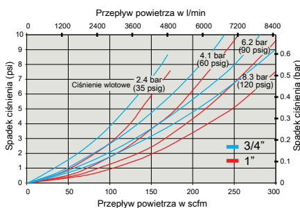
Filtr 3/4" & 1"
