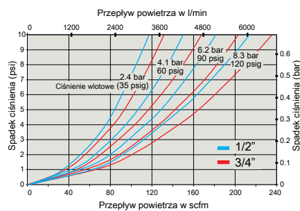
Filtr 1/2" & 3/4"
